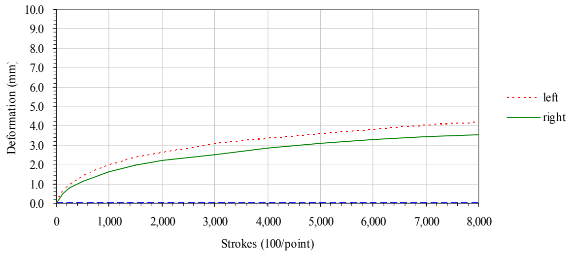
APA Rut Test
